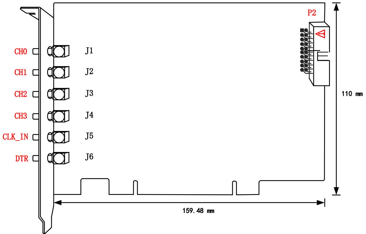
图 3-2-1 PCI-8514B/8504B 板卡尺寸图
