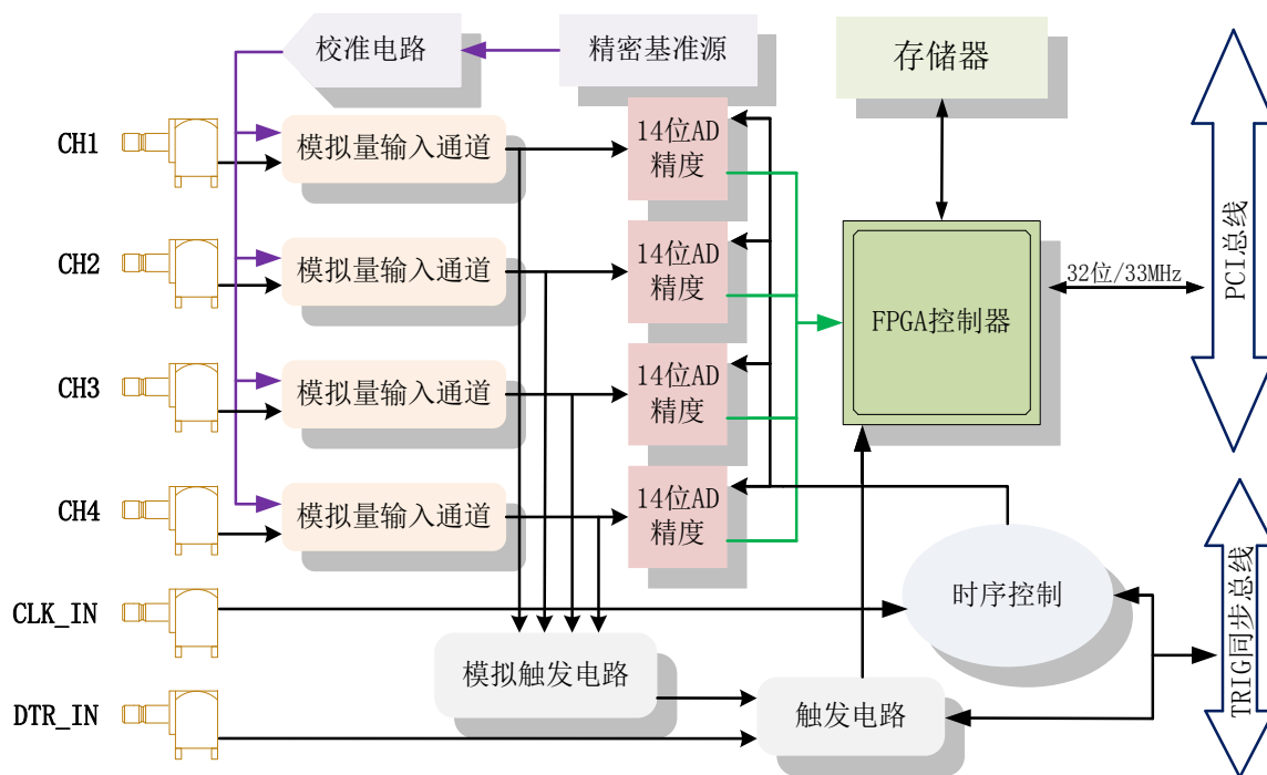
图 3-1-1 PCI8504B/8514B 系统框图
